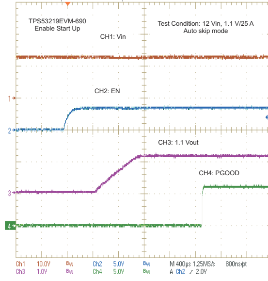
Figure 7-7. Enable Turn-On
